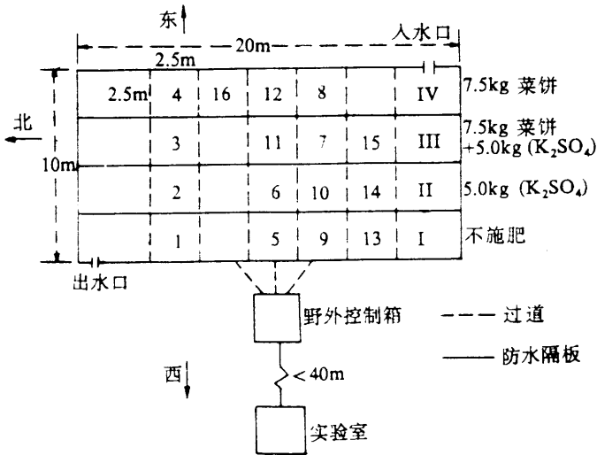
图 2 杭州稻田甲烷排放实验场地示意图
