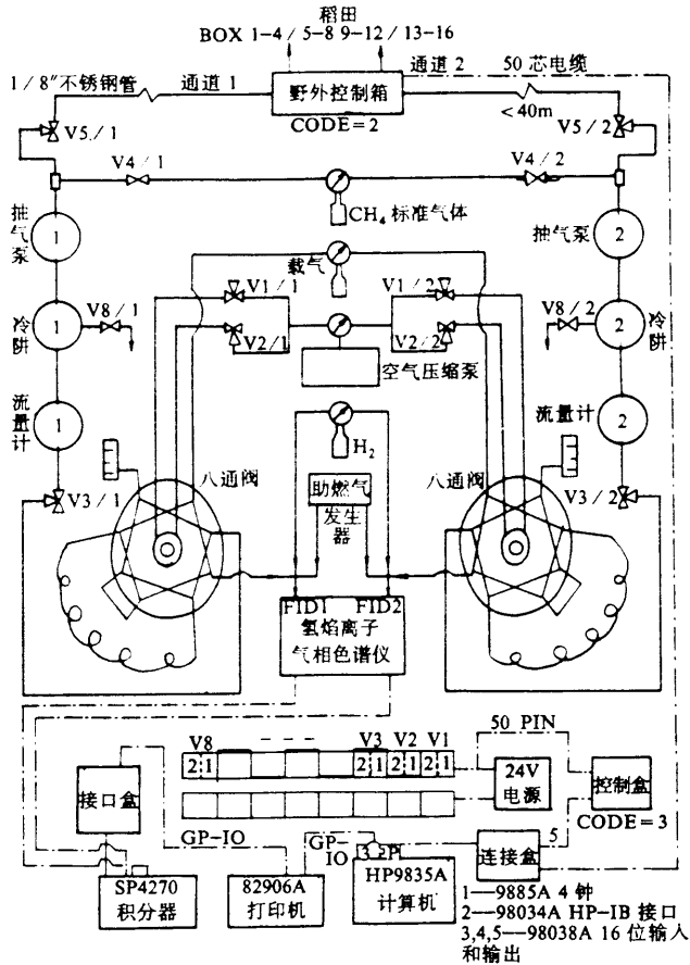
图 1 稻田甲烷排放自动连续的观测系统
