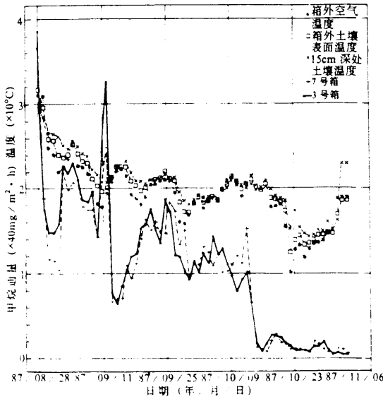
图 5 甲烷释放率与温度的关系
