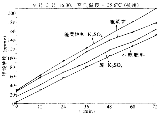
图 3 采集箱内甲烷浓度的线性上升
